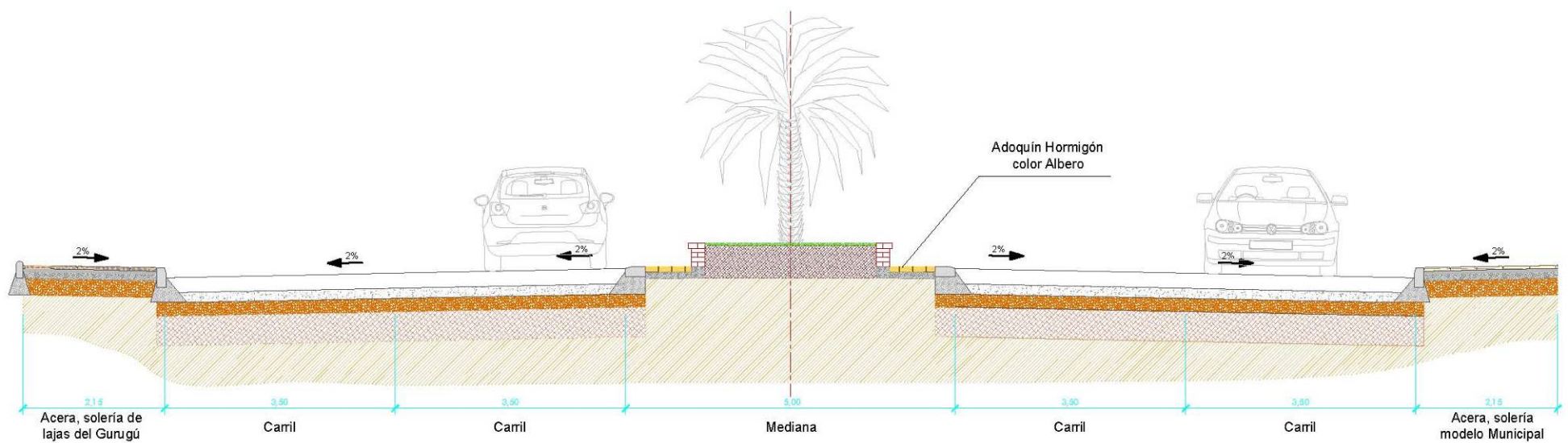
SECCIÓN TIPO DEL NUEVO VIAL DE CONEXIÓN ENTRE GLORIETAS
